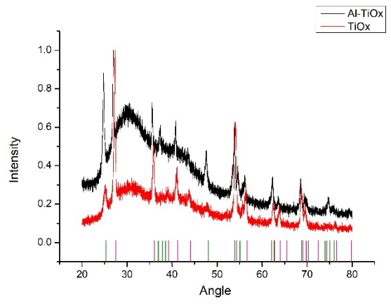
S4. XRD spectrum of TiOx
